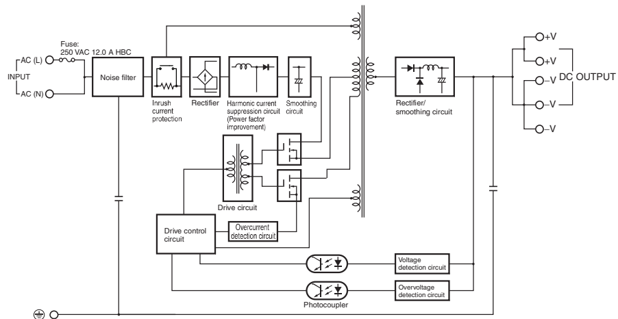
S8VK-C48024 (480W)
